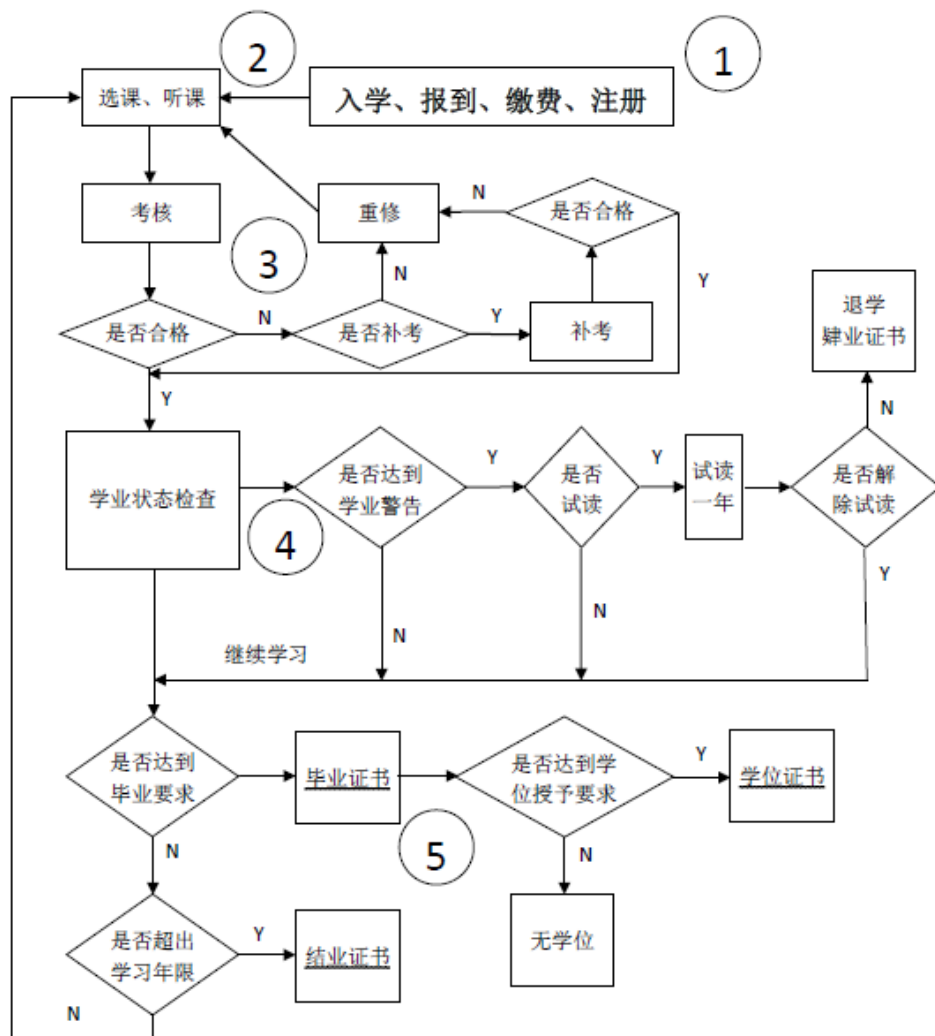
图 1 学习流程图
